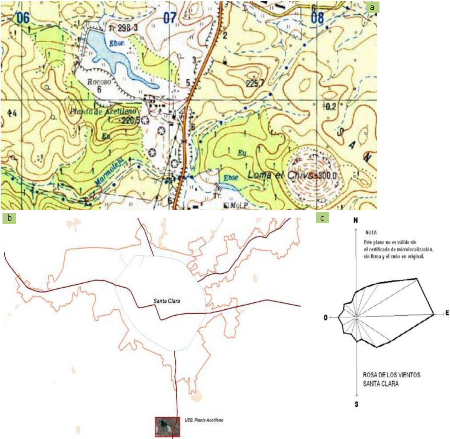
Figura 2a, b y c: 3 fotos correspondiente a la microlocalización de la Planta de Acetileno y rosa de los vientos de Santa Clara
