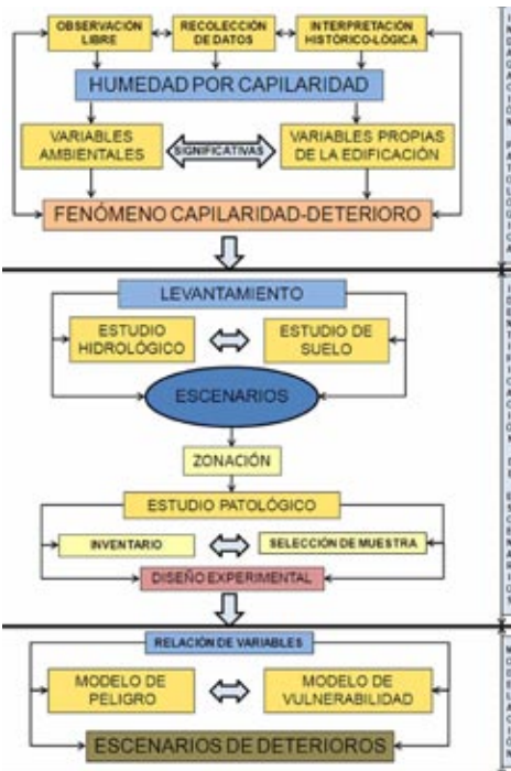
Figura 3: Esquema gráfico de las etapas que componen el proceso de modelación de la relación capilaridad-deterioro en edificaciones.
