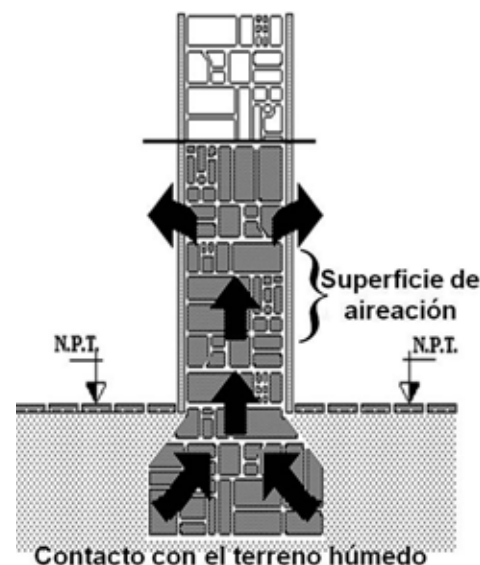
Figura 1: Esquema del movimiento del fenómeno de humedad por capilaridad en un elemento constructivo. Fuente: Pérez (2000).
