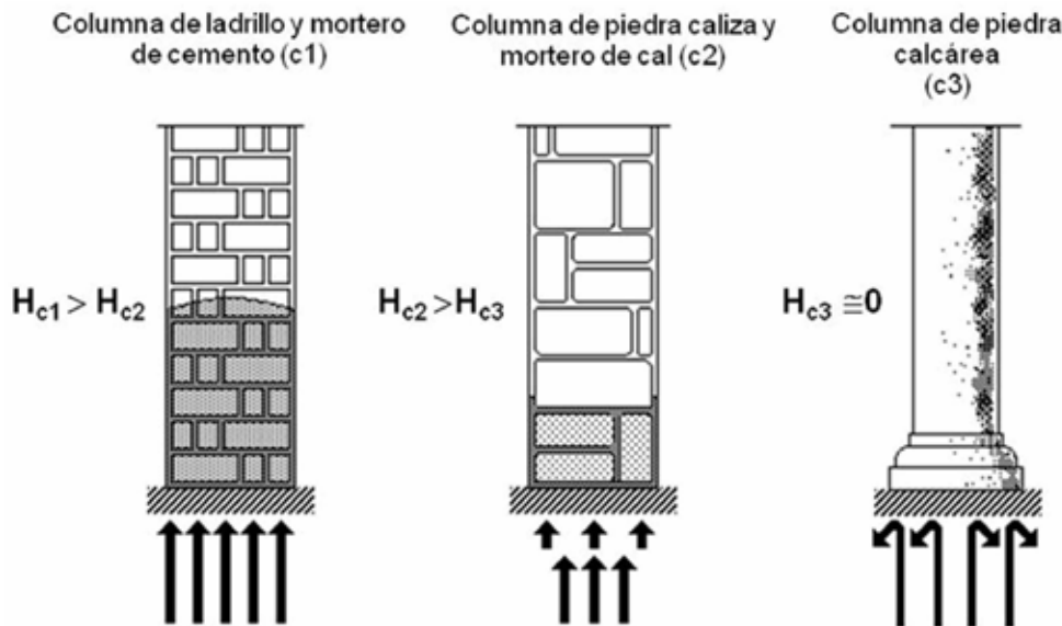
Figura 2: Esquemas que muestran el comportamiento de la altura capilar para diferentes tipos modulares de material de construcción. Fuente: Pérez (2000).
