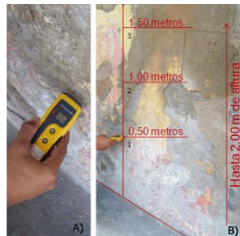
Figura 11. Fotos de: A) Equipo Surveymaster y B) Procedimiento de medición. Fuente: autores.
