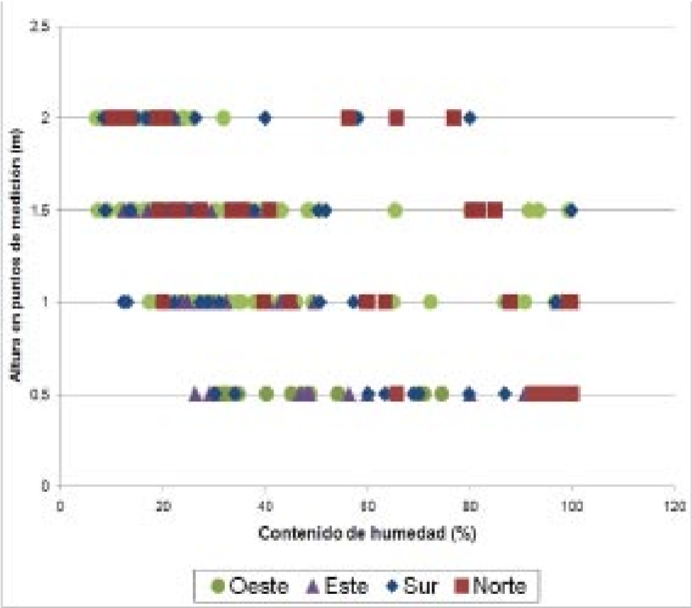
Figura 12. Gráfico con valores de contenido de la humedad en las fachadas según la orientación geográfica.
