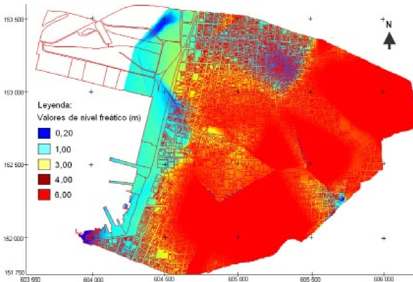
Figura 6. Modelo digital de la profundidad del nivel freático en el Centro Histórico santiaguero. Fuente: González et al , 2012.
