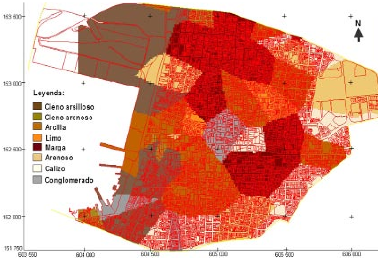
Figura 7. Mapa temático del tipo de suelo en el Centro Histórico santiaguero. Fuente: González et al , 2012.
