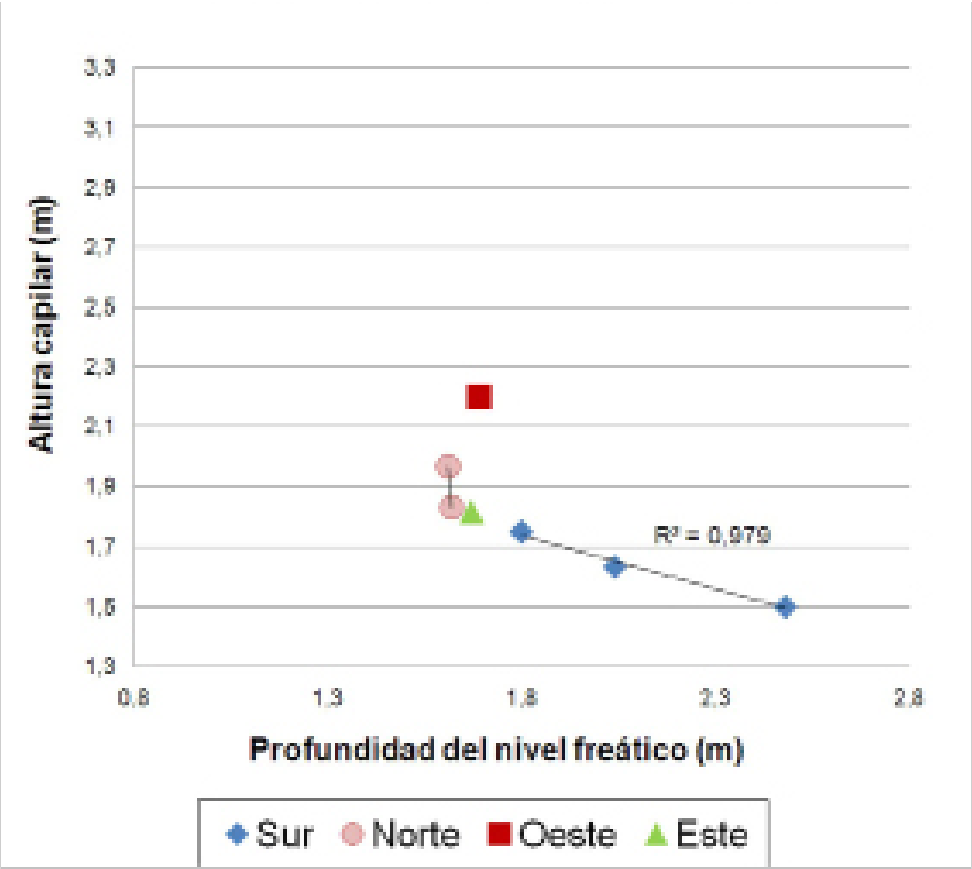
Figura 14. Tipo de suelo arena arcillosa.
