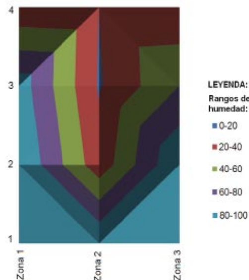
Figura 13. Distribución del contenido de humedad en la fachada del lote ubicado en la calle Gallo No. 364 y 362, según escala de colores.
