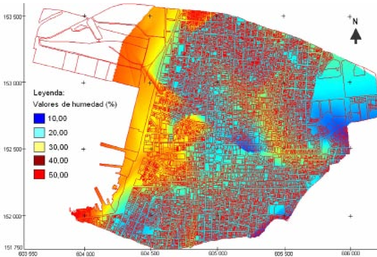
Figura 8. Modelo digital de humedad del suelo en el Centro Histórico santiaguero. Fuente: González, et al , 2012.
