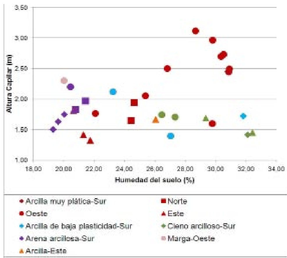
Figura 18: Gráfico que muestra la relación entre la altura capilar en fachadas y la humedad del suelo según el tipo de suelo.
