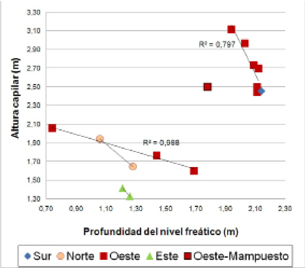
Figura 15. Tipo de suelo arcilla muy plástica.
