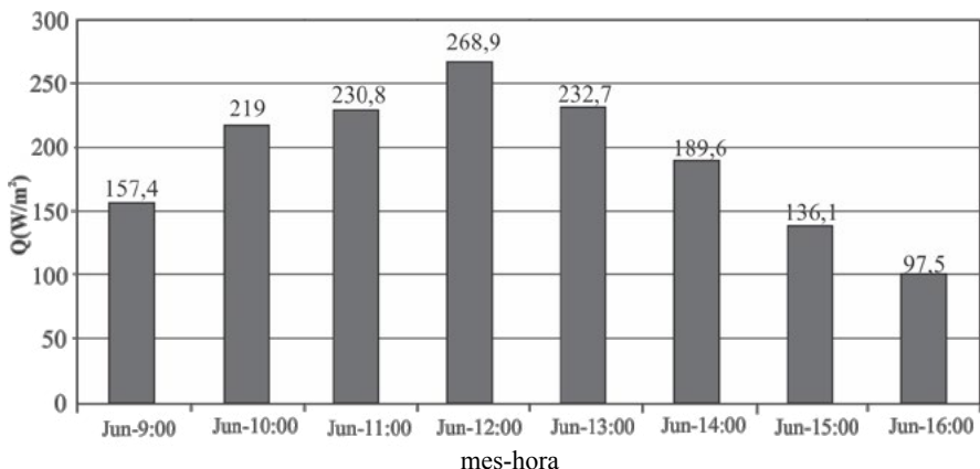
Figura 15: Flujo térmico por radiación solar ( W/m^2 ) que afecta el interior de un espacio debido al uso, en fachada norte, de una ventana de vidrio (1 400X1 200 mm), protegida por dos EPV (quebrasones con ángulo de 17°) cuyas dimensiones son: 1 300 mm de alto y 429 mm de vuelo.
